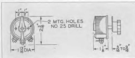
TYPE 301
