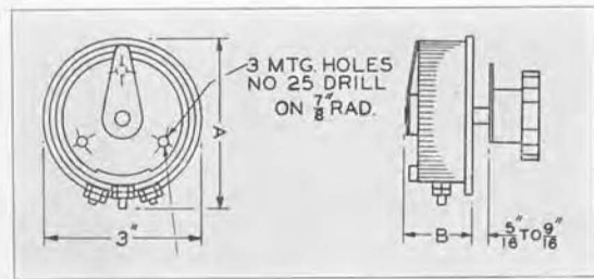
TYPE 301
